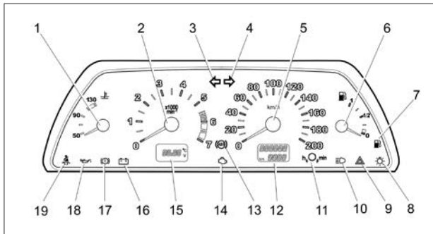
Рис. 14. Комбинация приборов
