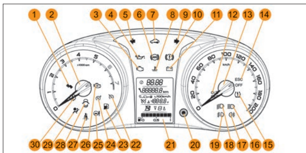
Рис. 29а. Комбинация приборов
