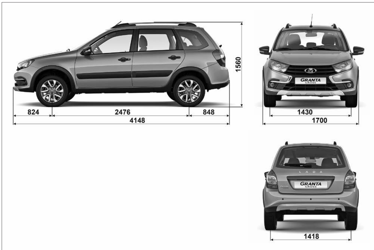
Рис. 62г. Габаритные (справочные) размеры автомобиля в модификации «Cross»
