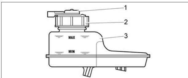
Рис. 46. Бачок гидропривода тормозов
