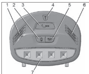
Рис. 18а. Блок освещения салона (в варианном исполнении)
