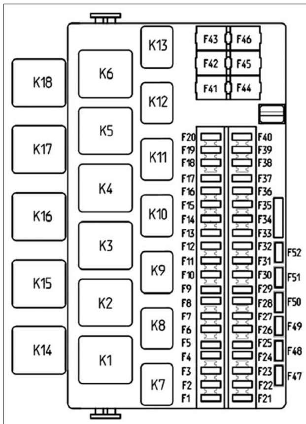
Рис. 54. Монтажный блок
