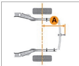
Схема размещения ТСУ (в варианном исполнении)
