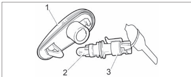
Рис. 57д. Боковой указатель поворота
