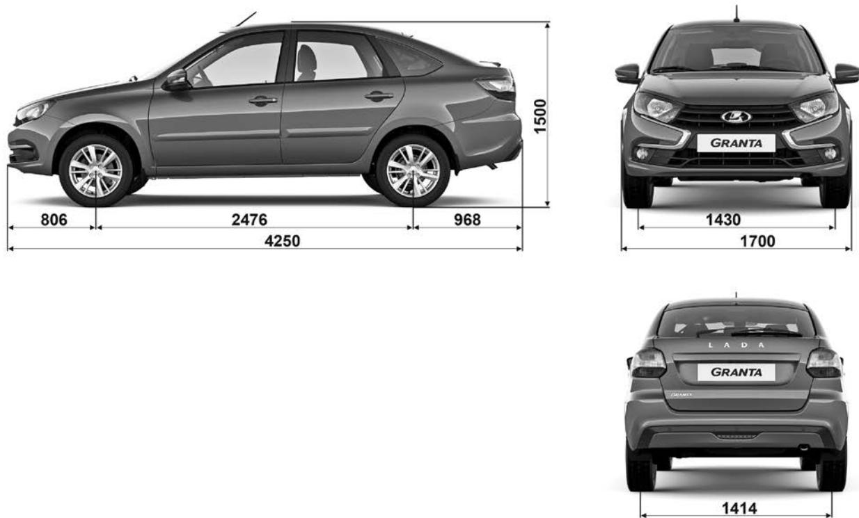
Рис. 626. Габаритные (справочные) размеры автомобиля с кузовом «лифтбек»
