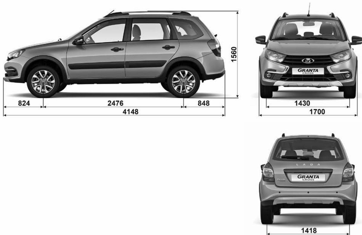
Рис. 62г. Габаритные (справочные) размеры автомобиля в модификации «Cross»
