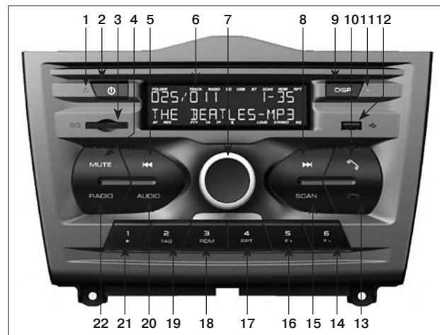
Рисунок 1. Внешний вид и форма лицевой панели радиоприемника
