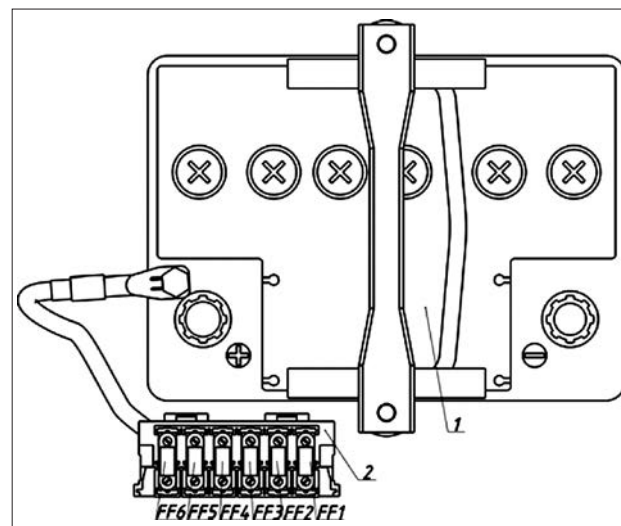
Рис. 55. Блок предохранителей моторного отсека
