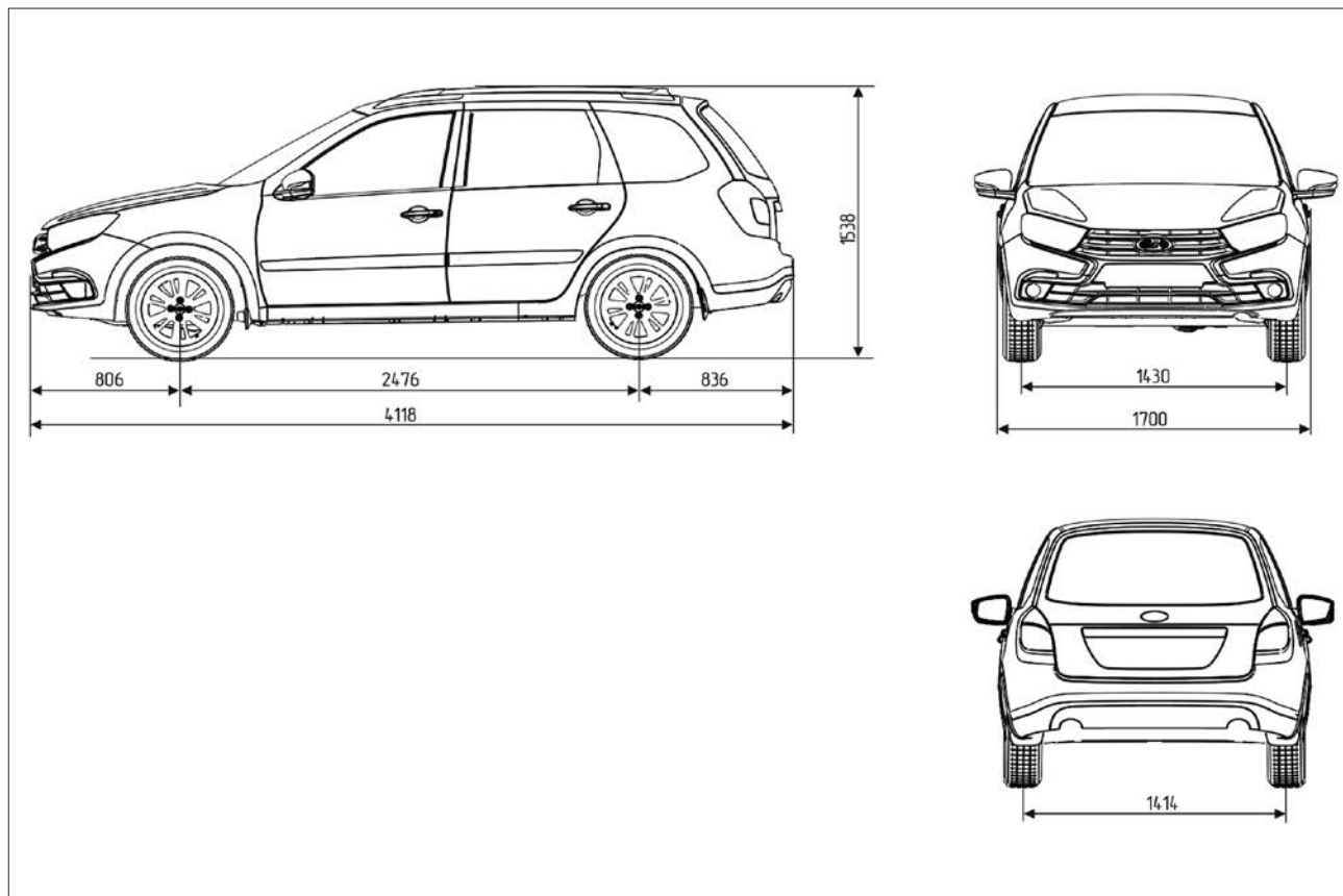
Рис. 62в. Габаритные (справочные) размеры автомобиля с кузовом «универсал»
