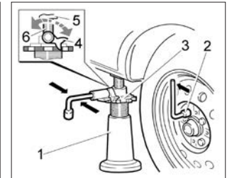
Рис. 50б. Подъем автомобиля при замене колес
