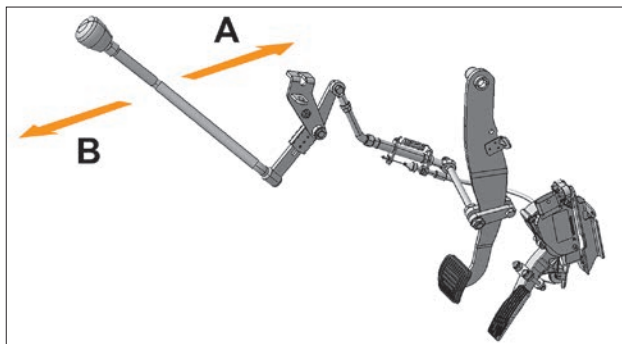
Рис. 2. Устройство ручного управления педалями акселератора и тормоза для автомобилей с автоматической (АКП) коробкой передач и левым расположением органов управления:
