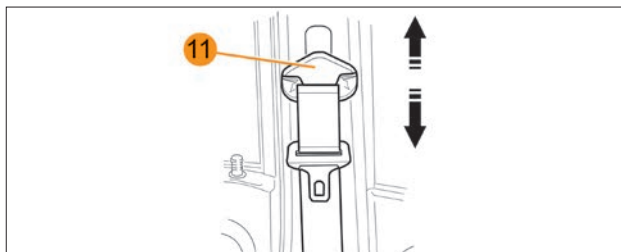
Рис. 13д. Регулировка ремня безопасности (в варианном исполнении)
