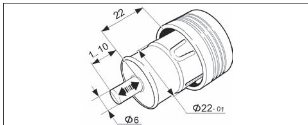
Рис. 21б. Размеры вилки электрического прибора для использования в патроне для подключения дополнительных потребителей
