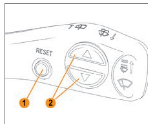
Рис. 29в. Переключатель стеклоочистителя с 3-мя клавишами управления
