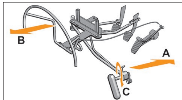
Рис. 1. Устройство ручного управления педалями акселератора, тормоза и сцепления для автомобилей с механической коробкой передач (МКП) и правым расположением органов управления:
