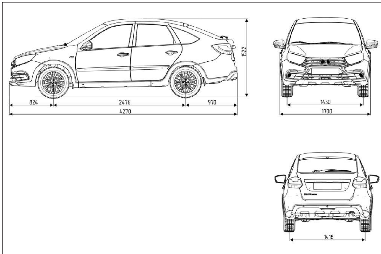
Рис. 62д. Габаритные (справочные) размеры автомобиля в модификации «лифтбек Cross»
