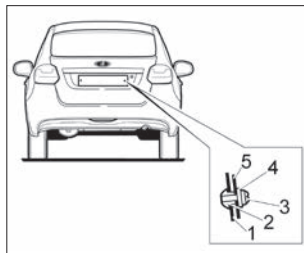
Рис. 41а. Крепление заднего номерного знака
