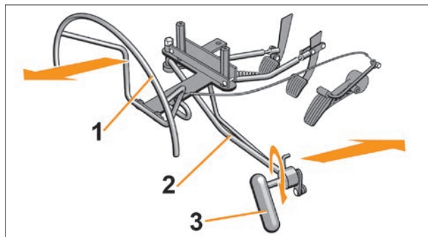
Рис. 3. Устройство ручного управления педалями акселератора, тормоза и сцепления для автомобилей с механической коробкой передач (МКП) и правым расположением органов управления:
