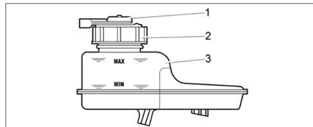
Рис. 46. Бачок гидропривода тормозов
