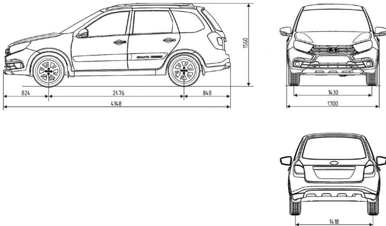
Рис. 62г. Габаритные (справочные) размеры автомобиля в модификации «универсал Cross»
