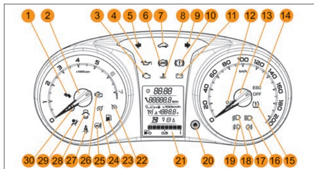
Рис. 29а. Комбинация приборов
