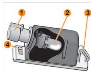
Рис. 58а. Фонарь освещения номерного знака
