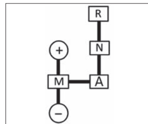
Рис. 36г. Схема переключения передач
