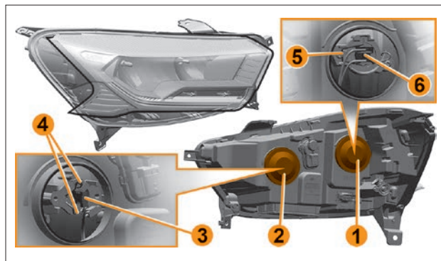
Рис. 6.12.1. Замена ламп ближнего и дальнего света в блок-фаре
