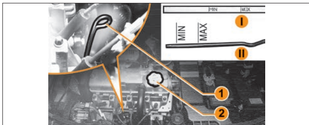
Рис. 6.3.1. Масляный щуп двигателя (в вариантном исполнении)
