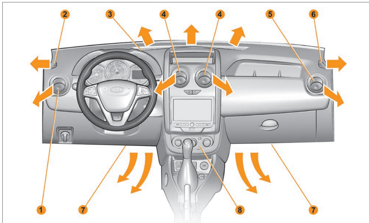
Рис. 3.12.1. Климатическая система (в варианном исполнении)
