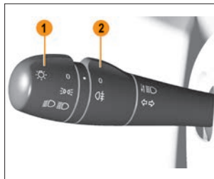
Рис. 3.9.2. Кольца управления на левом рычаге подрулевого переключателя (в варианном исполнении)
