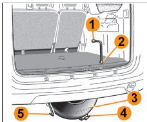
Рис. 6.9.1. Снятие запасного колеса
