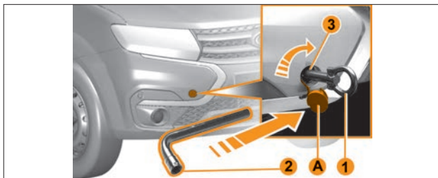
Рис. 6.14.1. Передняя вворачиваемая буксирная проушина
