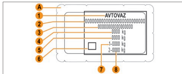
Рис. 7.1.2. Табличка изготовителя (в варианном исполнении)
