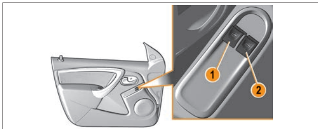
Рис. 4.1.2. Блок управления электростеклоподъемниками А (в варианном исполнении)
