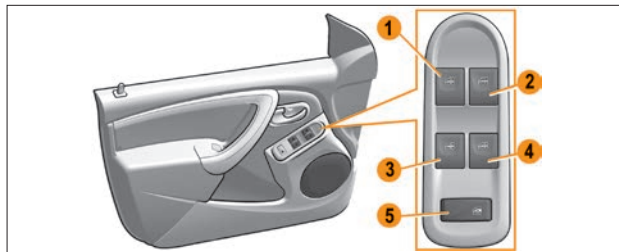
Рис. 4.1.3. Блок управления электростеклоподъемниками В (в варианном исполнении)
