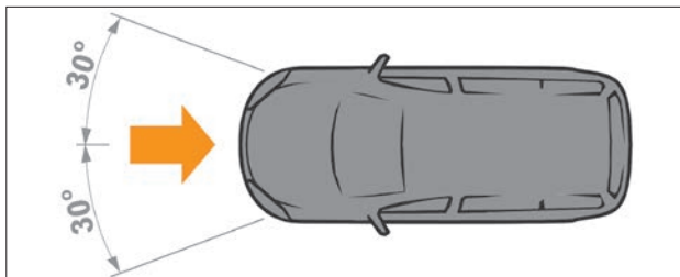
Рис. 2.6.5. Зона действия и срабатывания фронтальных подушек безопасности
