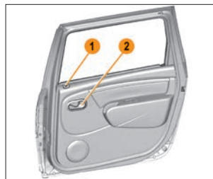
Рис. 1.4.3. Открытие задних дверей изнутри (в варианном исполнении)
