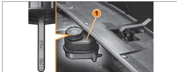
Рис. 6.7.1. Бачок гидроусилителя рулевого управления
