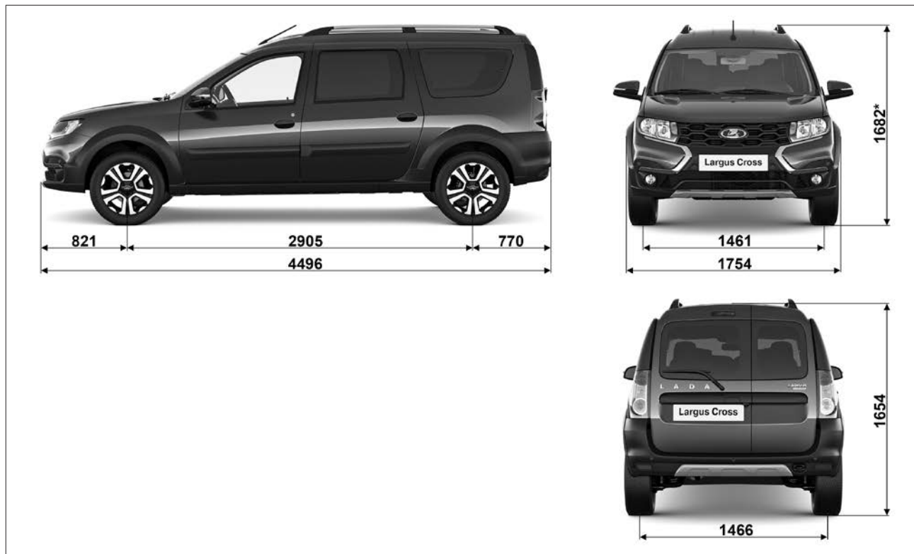
Рис. 7.2.3. Габаритные (справочные) размеры автомобиля Largus Cross (в вариантном исполнении)
