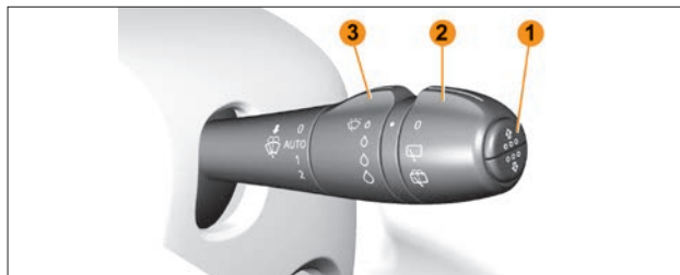
Рис. 3.9.8. Кольца и кнопки управления на правом рычаге подрулевого переключателя (в варианном исполнении)
