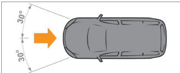
Рис. 2.6.5. Зона действия и срабатывания фронтальных подушек безопасности
