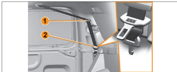
Рис. 2.5.6б. Фиксация среднего ремня безопасности (в варианном исполнении)
