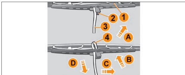
Рис. 6.8.2. Замена щеток стеклоочистителя ветрового стекла (в варианном исполнении)
