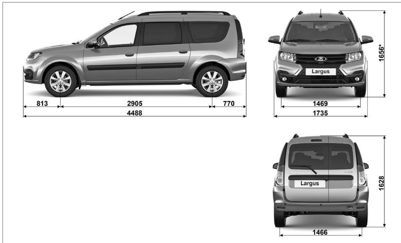
Рис. 7.2.1. Габаритные (справочные) размеры автомобиля Largus «универсал» (в варианном исполнении)
