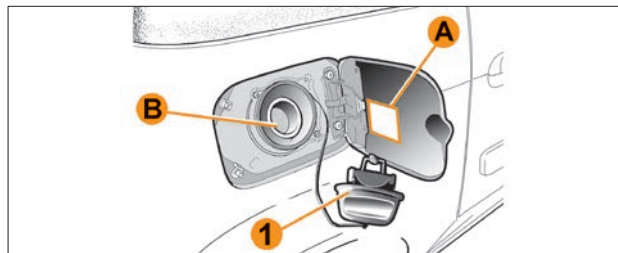
Рис. 5.17.1. Пробка наливной трубы топливного бака
