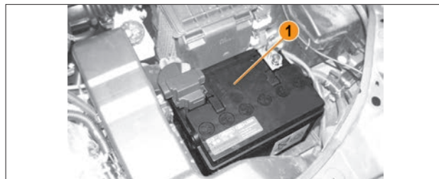
Рис. 6.10.1. Аккумуляторная батарея
