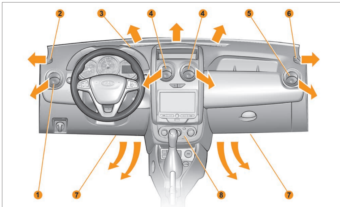
Рис. 3.12.1. Климатическая система (в варианном исполнении)
