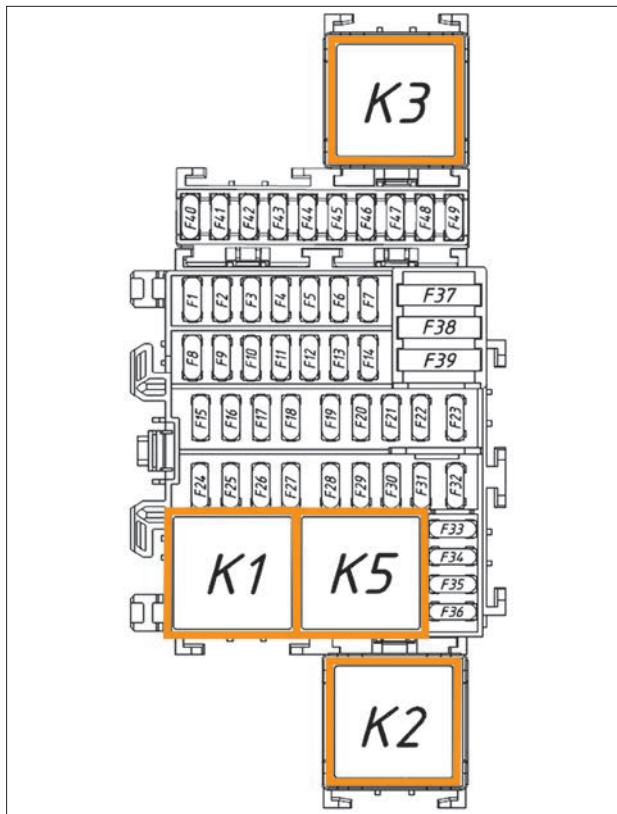
Рис. 8.4.1. Схема расположения предохранителей и реле в монтажном блоке салона (в варианном исполнении)
