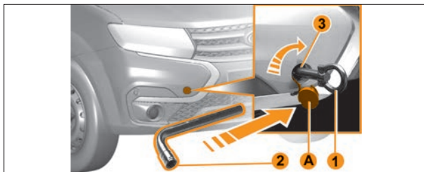
Рис. 6.14.1. Передняя вворачиваемая буксирная проушина
