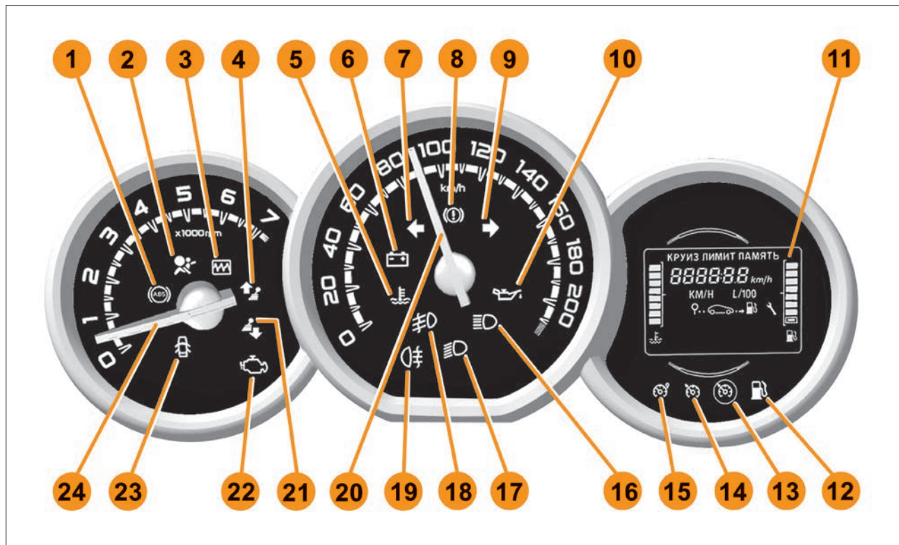
Рис. 3.2.1. Комбинация приборов (в варианном исполнении)
