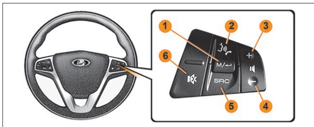
Рис. 4.6.2. Блок управления MMC LADA EnjoY Pro (в варианном исполнении)
