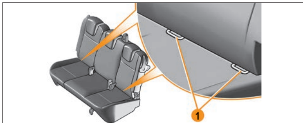
Рис. 2.8.4. Кронштейны нижних креплений ISOFIX (в варианном исполнении)
