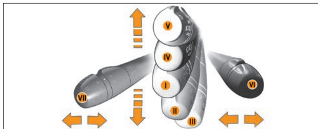
Рис. 3.9.4. Положения левого рычага подрулевого переключателя (в варианном исполнении)
