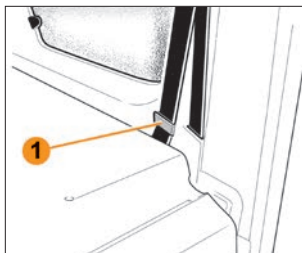
Рис. 2.5.5. Фиксация бокового ремня безопасности
