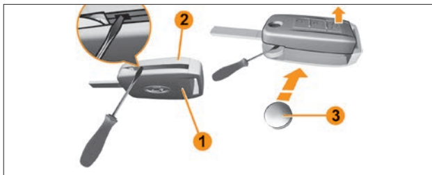
Рис. 6.11.16. Замена элемента питания в ПДУ (в варианном исполнении)
