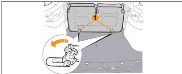
Рис. 2.3.5. Защелки крепления сиденья третьего ряда
