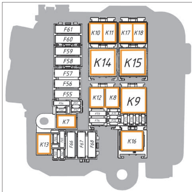
Рис. 8.4.2. Схема расположения предохранителей и реле в монтажном блоке моторного отсека (в вариантном исполнении)
