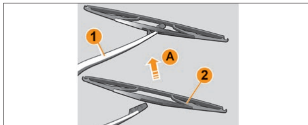
Рис. 6.8.3. Замена щетки стеклоочистителя заднего стекла (в варианном исполнении)
