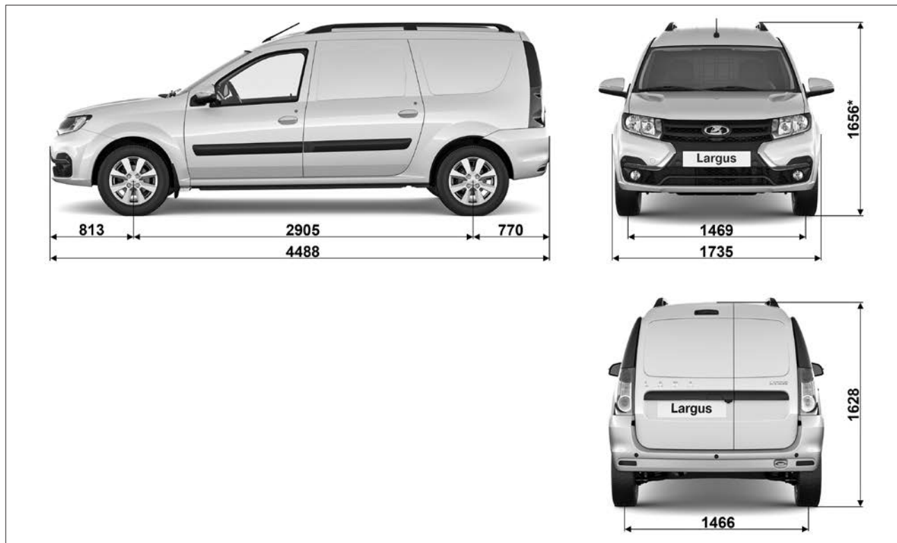
Рис. 7.2.2. Габаритные (справочные) размеры автомобиля Largus «фургон» (в варианном исполнении)
