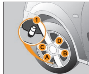
Рис. 6.9.2. Снятие и установка декоративного колпака (в варианном исполнении)
