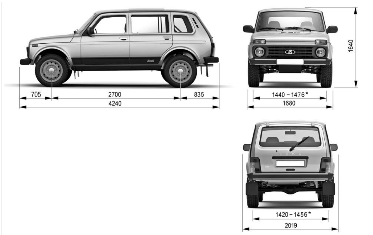
Рис. 51. Габаритные размеры автомобиля LADA Niva Legend (5 дверей)
