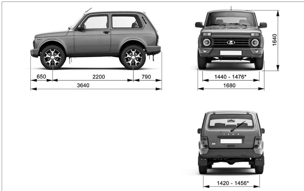
Рис. 52. Габаритные размеры автомобиля LADA Niva Legend Urban (3 двери)
