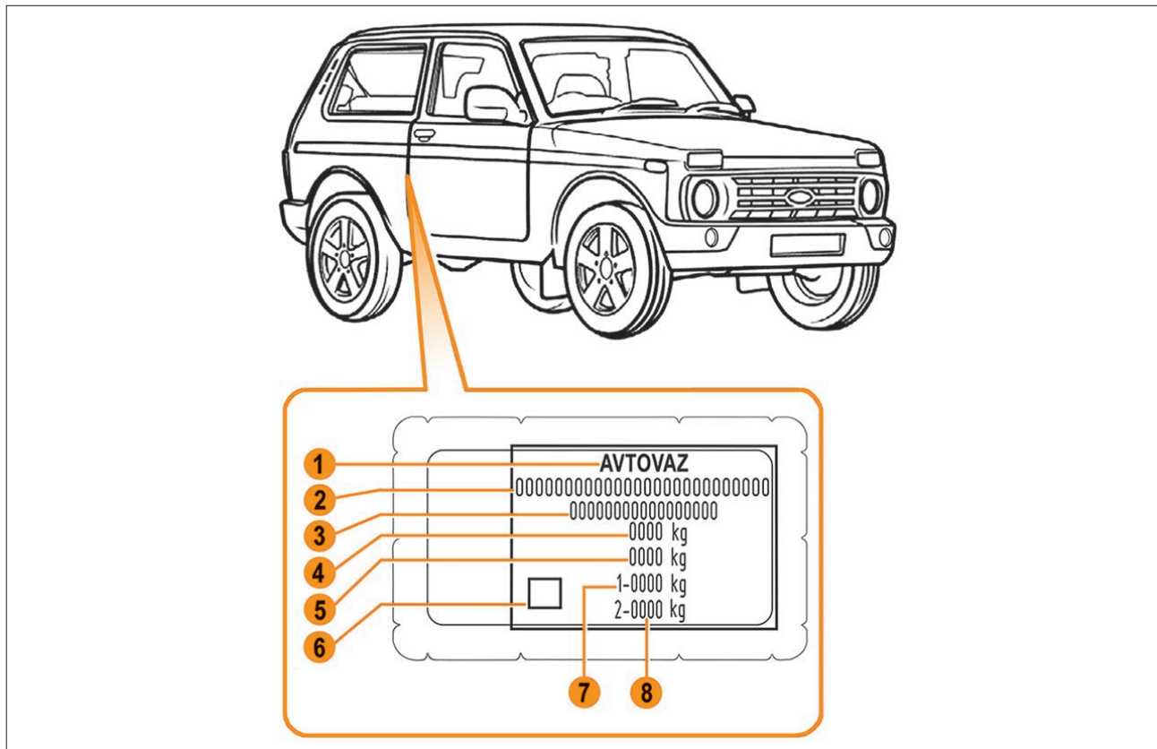
Рис. 54. Табличка изготовителя (в варианном исполнении)
