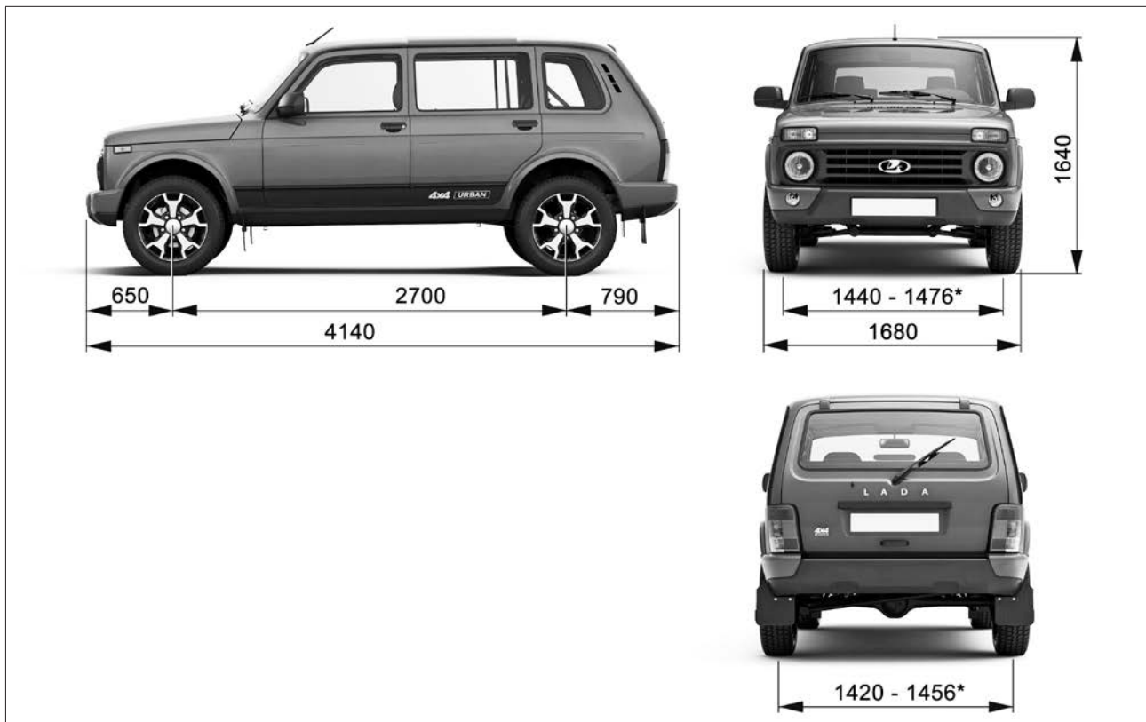
Рис. 53. Габаритные размеры автомобиля LADA Niva Legend Urban (5 дверей)
