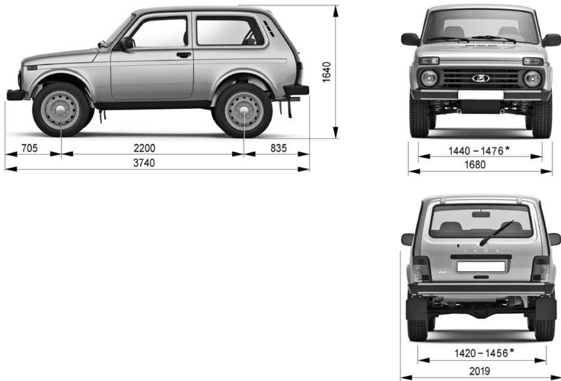
Рис. 50. Габаритные размеры автомобиля LADA Niva Legend (3 двери)
