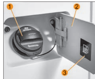
Рис. 5. Пробка топливного бака
