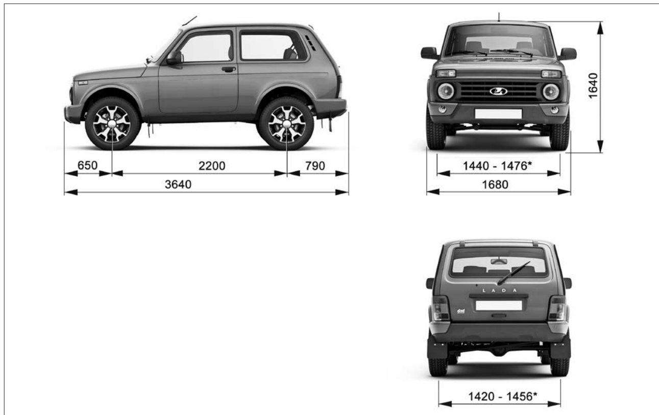
Рис. 51. Габаритные размеры автомобиля LADA Niva Legend Urban (3 двери)
