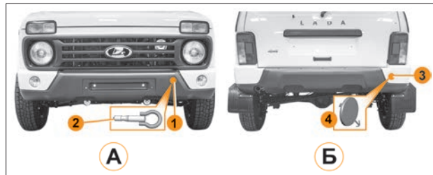
Рис. 33. Расположение вворачиваемых буксирных проушин (в варианном исполнении)
