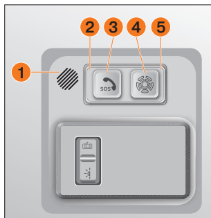
Рис. 70а. Компоненты БИП
