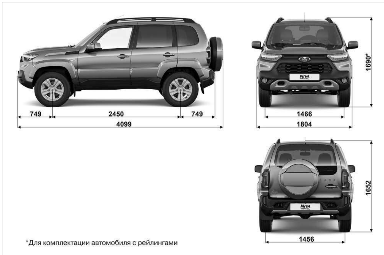
Рис. 87. Габаритные (справочные) размеры автомобиля (в варианном исполнении)
