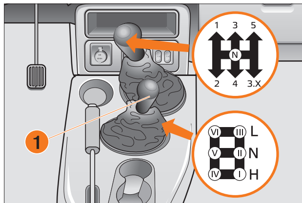
Рис. 48. Положение рычагов трансмиссии
