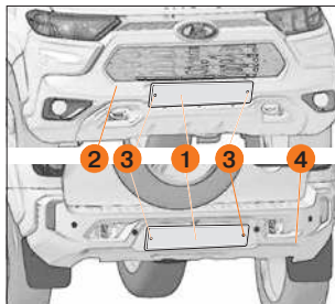
Рис. 63. Крепление номерных знаков
