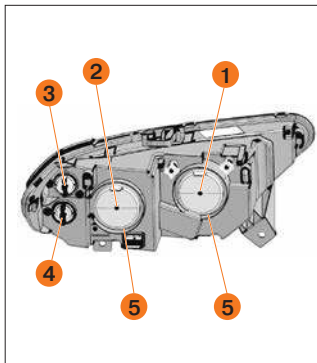
Рис. 82. Блок-фара
