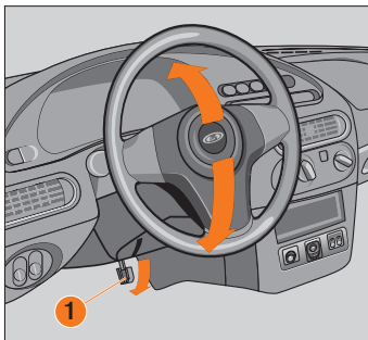
Рис. 6д. Рукоятка регулировки положения рулевой колонки
