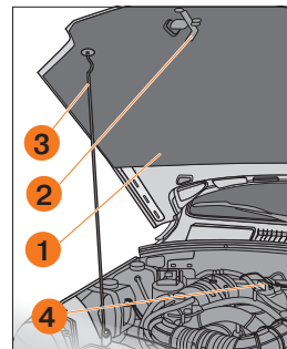
Рис. 37. Открывание капота
