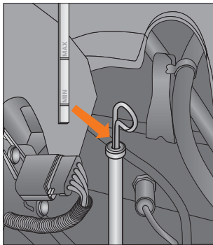
Рис. 71. Проверка уровня масла в картере двигателя
