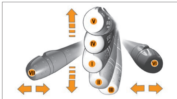
Рис. 3.9.3. Положения левого рычага подрулевого переключателя (в варианном исполнении)
