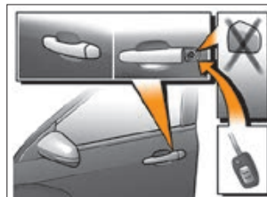
Рис. 1.3.1. Механическая разблокировка/блокировка замка двери водителя
