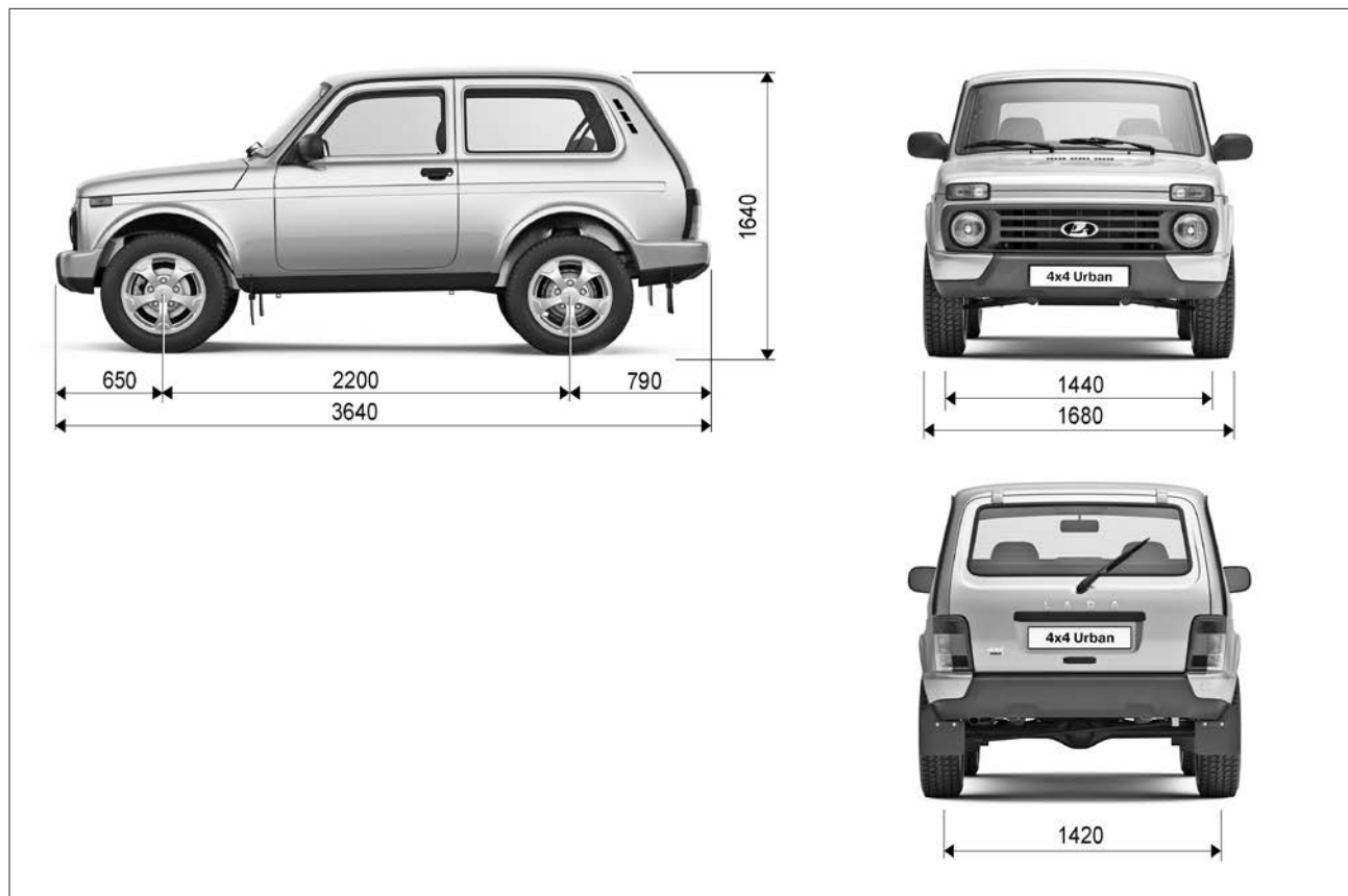
Рис.32. Габаритные размеры автомобиля LADA 4x4 Urban 3 дв.
