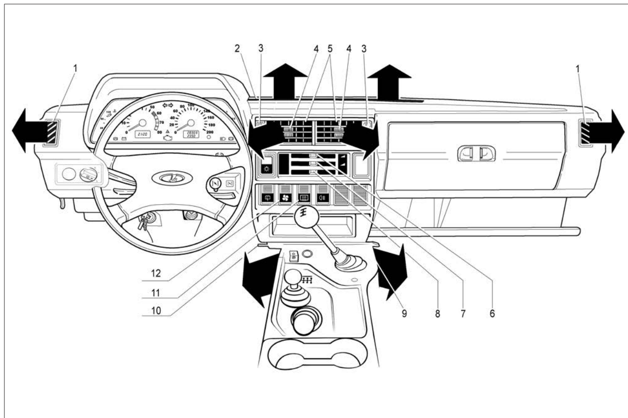
Рис. 23. Органы управления вентиляцией и отоплением салона
