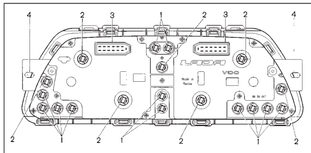
Рис. 48. Комбинация приборов
