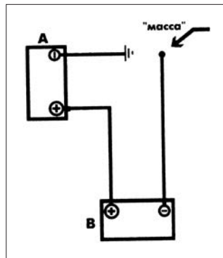
Рис. 22. Схема подключения вспомогательной батареи
