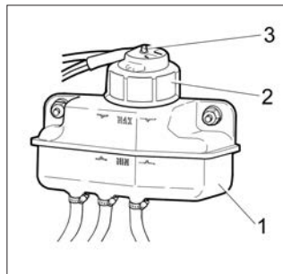
Рис. 35. Бачок гидропривода тормозов и сцепления
