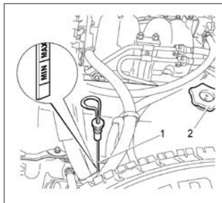
Рис. 33. Проверка уровня масла в картере двигателя
