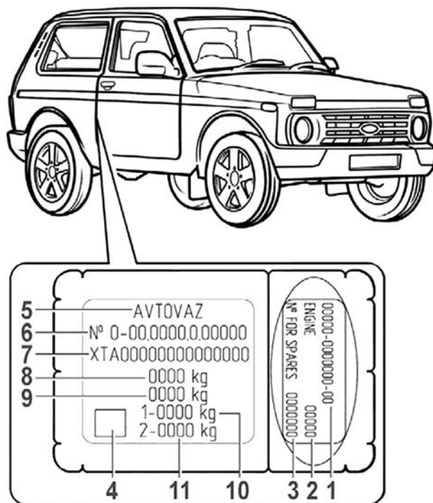
Рис. 54. Паспортные данные.
