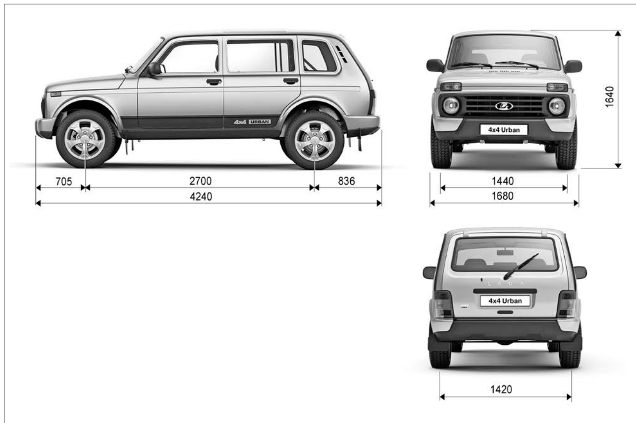
Рис. 53. Габаритные размеры автомобиля LADA 4x4 Urban 5 дв.
