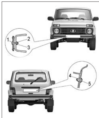
Рис. 16. Установка номерных знаков
