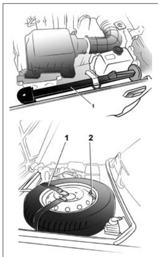
Рис. 43. Укладка и крепление домкрата и запасного колеса
