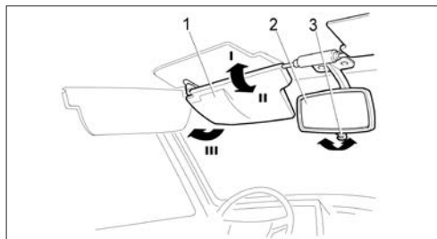
Рис. 10. Противосолнечные козырьки и зеркала
