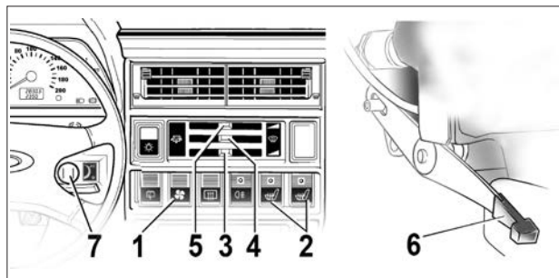
Рис. 24. Органы управления климатической установкой
