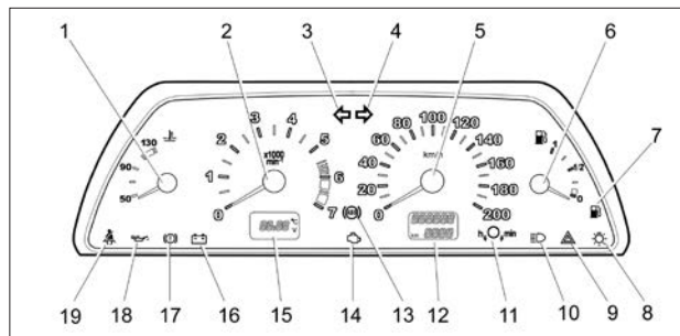
Рис. 13. Комбинация приборов
