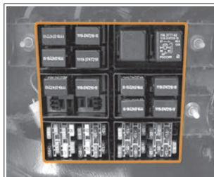
Рис. 48. Монтажный блок в салоне
