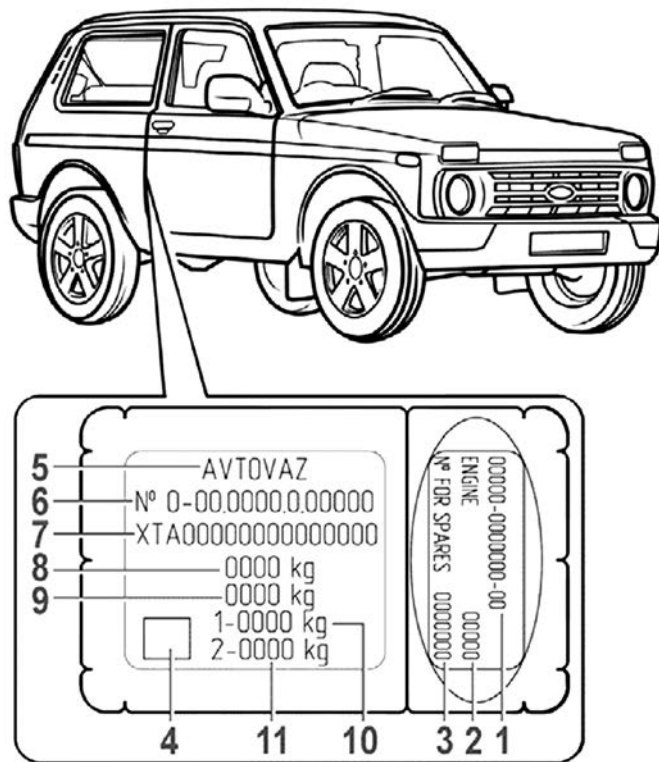
Рис. 59. Паспортные данные. Место установки таблички: 21214 – панель боковины правой; 2131 – панель боковины средней правой
