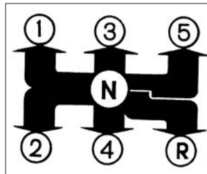
Рис. 23. Схема переключения передач
