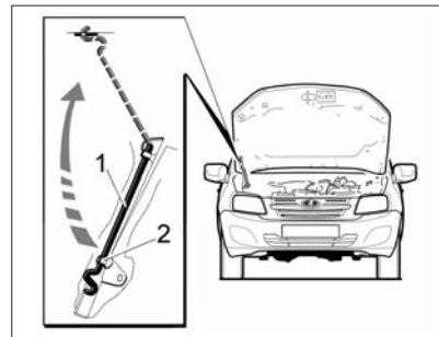
Рис. 24. Открывание капота
