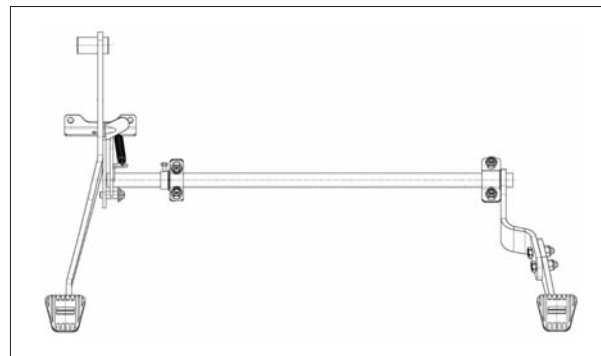
Схема для автоматической коробки передач
