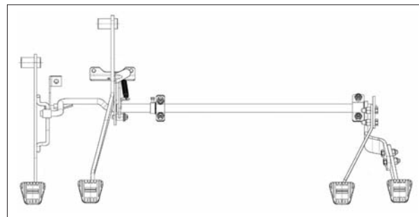
Схема для механической коробки передач
