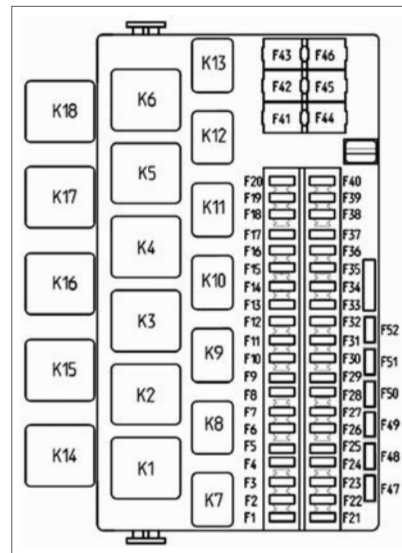
Рис. 57. Монтажный блок
