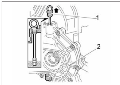
Рис. 45б. Проверка уровня масла в коробке передач
