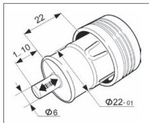
Рис. 216. Размеры вилки электрического прибора для использования в патроне для подключения дополнительных потребителей
