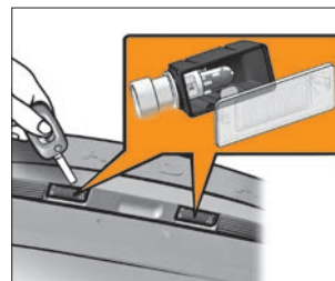
Рис. 58б. Посадочное место фонаря освещения номерного знака
