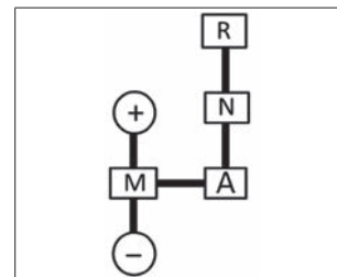
Рис. 36г. Схема переключения передач
