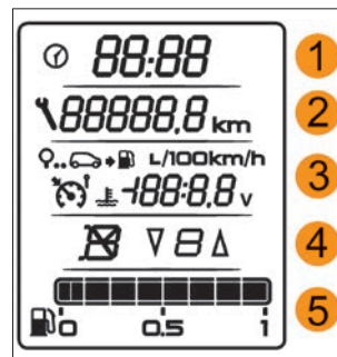
Рис. 29б. Жидкокристаллический дисплей
