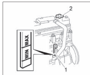
Рис. 44. Проверка уровня масла в картере двигателя 8-клапанного двигателя
