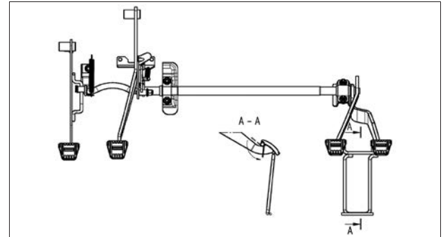
Схема для механической коробки передач
