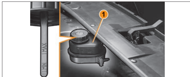
Рис. 6.7.1. Бачок гидроусилителя рулевого управления (в варианном исполнении)
