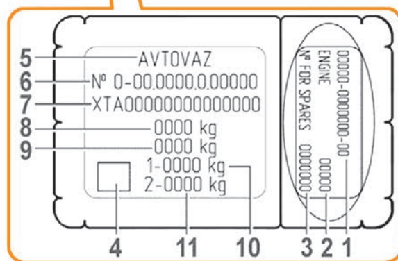
Рис. 56. Паспортные данные. Место установки таблички: LADA Niva Legend 3 дв. – панель боковины правой; LADA Niva Legend 5 дв. – панель боковины средней правой
