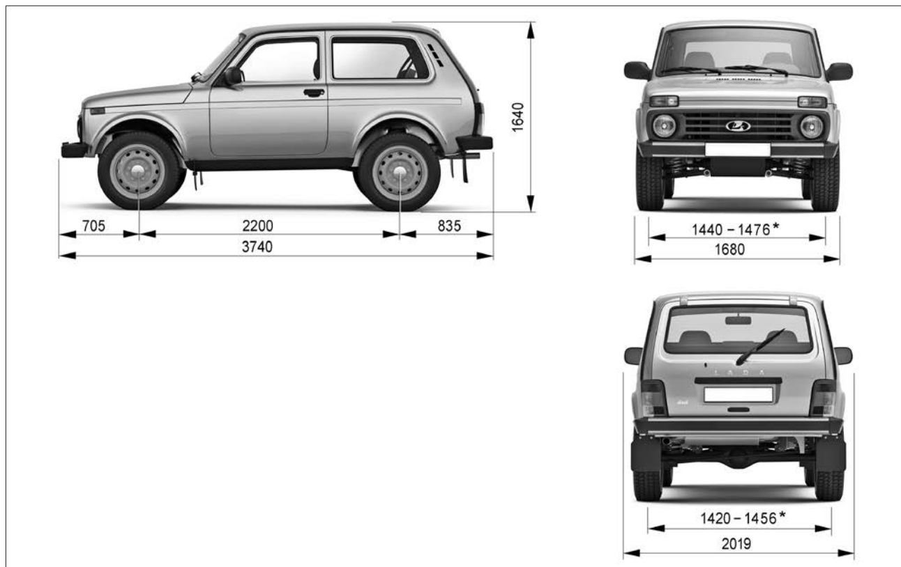
Рис. 52. Габаритные размеры автомобиля LADA Niva Legend 3 дв.
