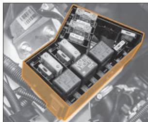
Рис. 49. Монтажный блок в моторном отсеке
