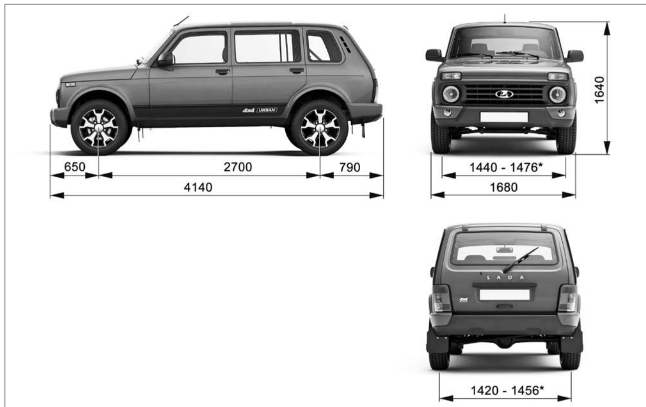
Рис. 55. Габаритные размеры автомобиля LADA Niva Legend Urban 5 дв.
