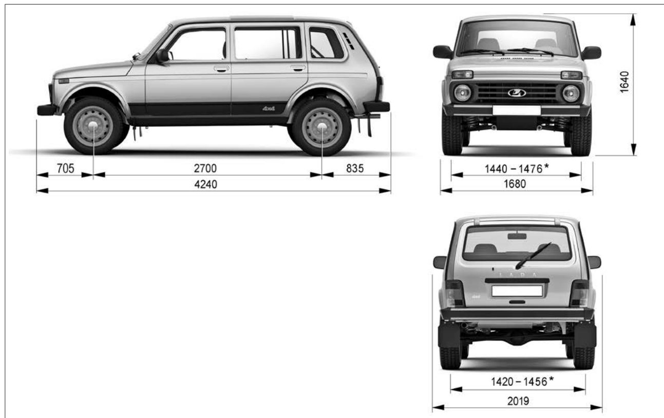
Рис. 53. Габаритные размеры автомобиля LADA Niva Legend 5 дв.
