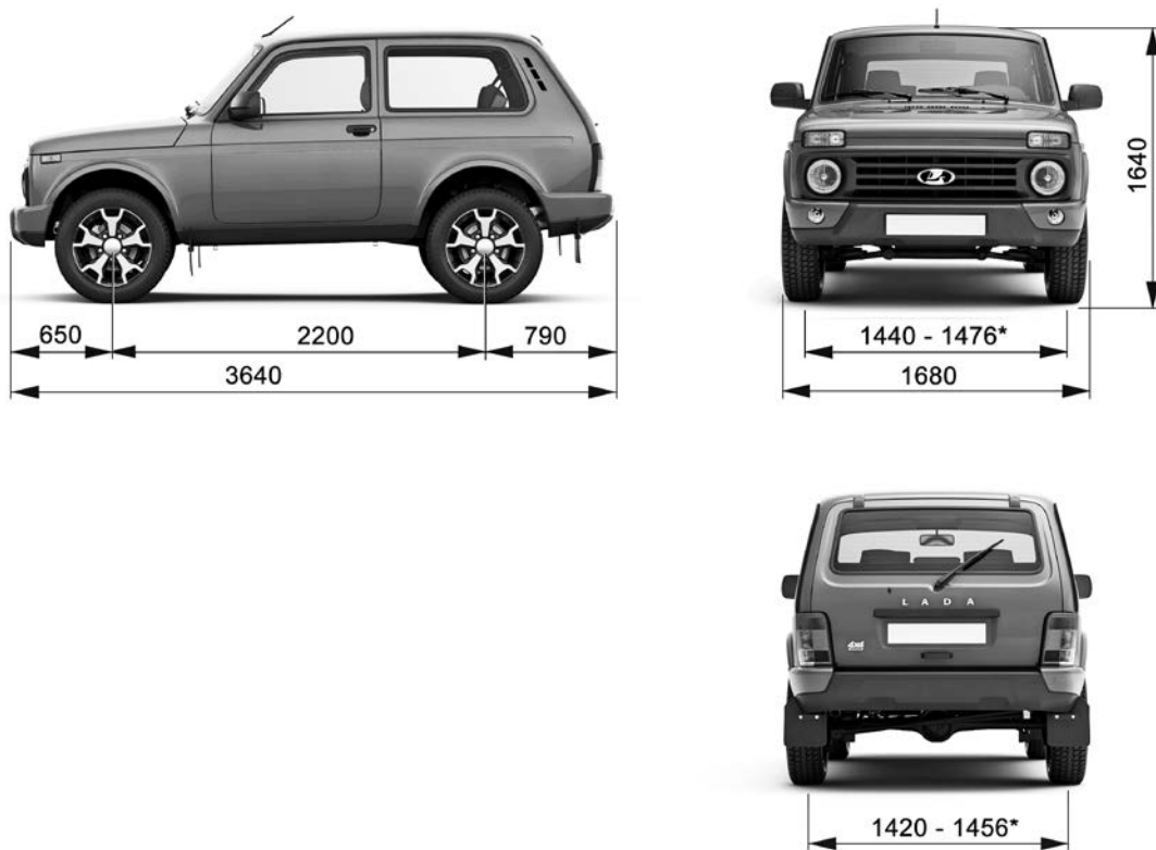
Рис. 54. Габаритные размеры автомобиля LADA Niva Legend Urban 3 дв.
