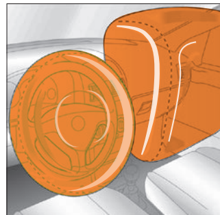
Рис. 16. Система надувных подушек безопасности (в варианте исполнения)
