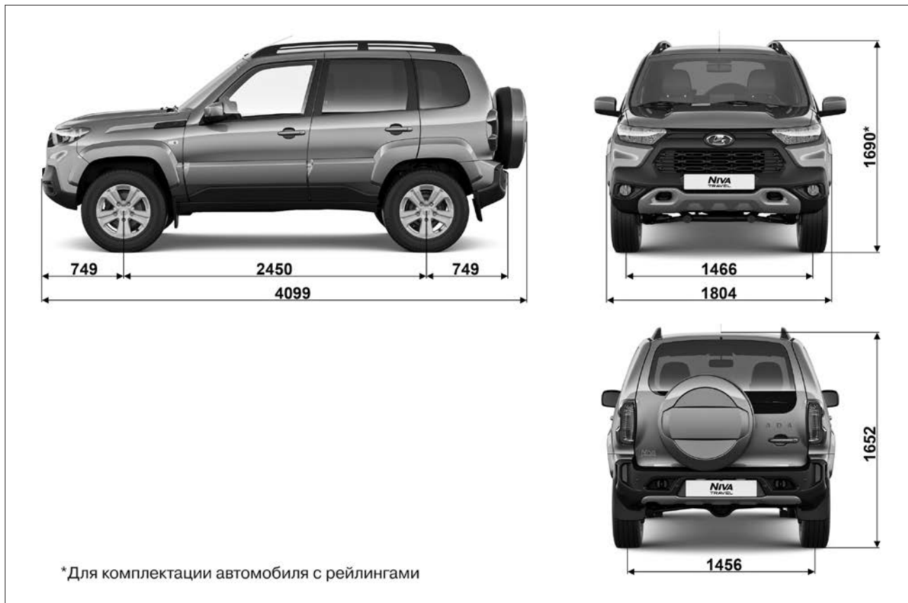
Рис. 90. Габаритные (справочные) размеры автомобиля (в варианном исполнении)
