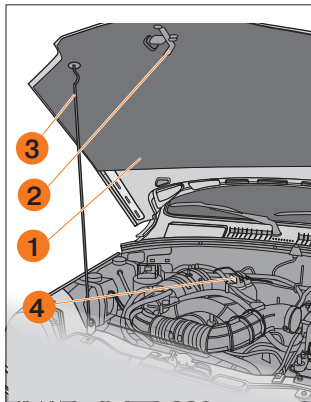
Рис. 37. Открывание капота
