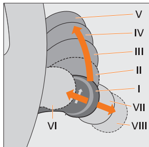
Рис. 45. Подрулевые переключатели
