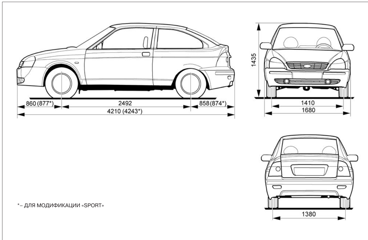
Рис. 96. Габаритные и справочные размеры автомобиля LADA 2172 Coupe
