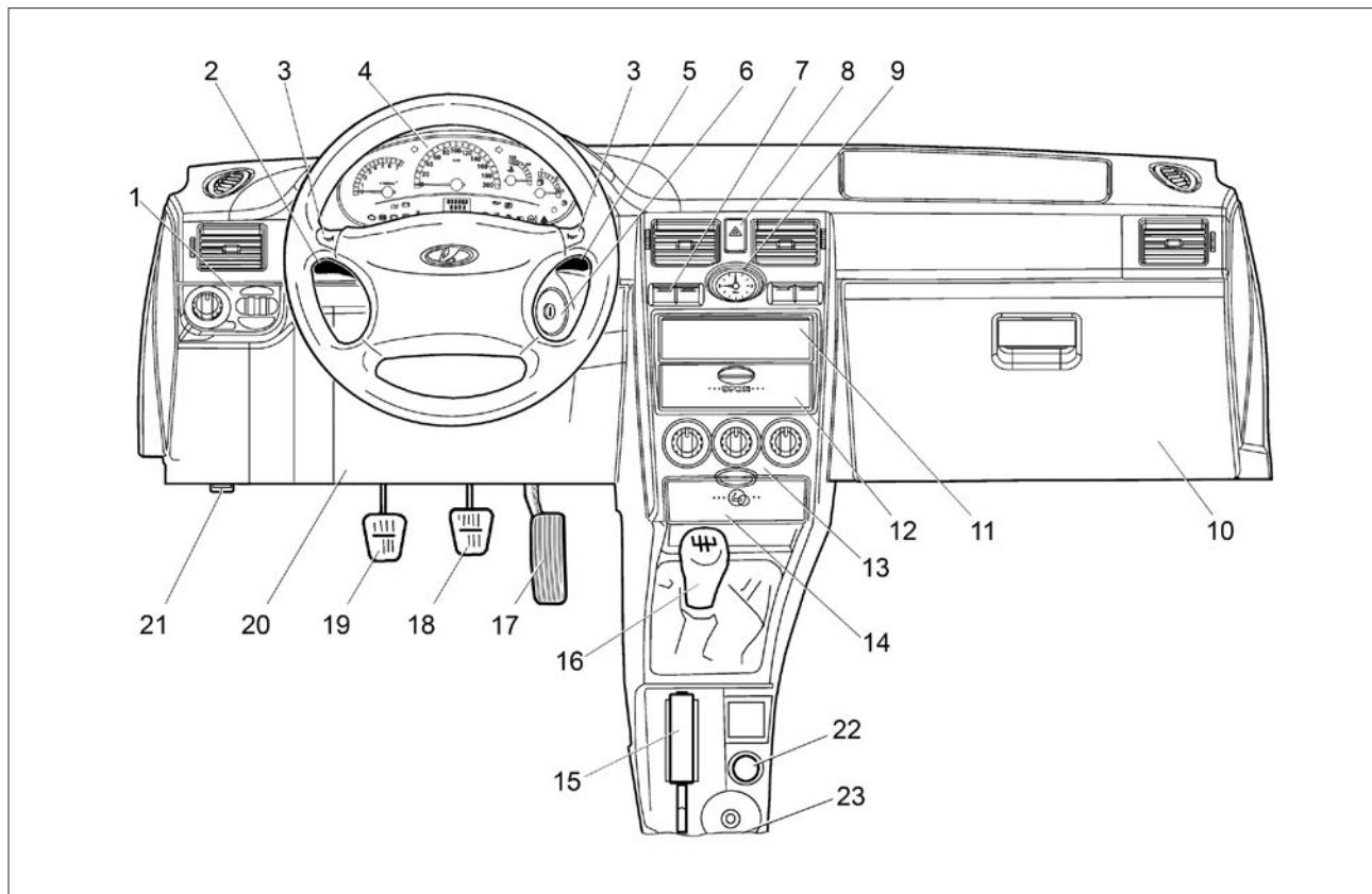
Рис. 38. Органы управления и приборы
