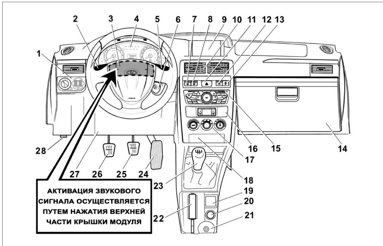
Рис. 40. Органы управления и приборы
