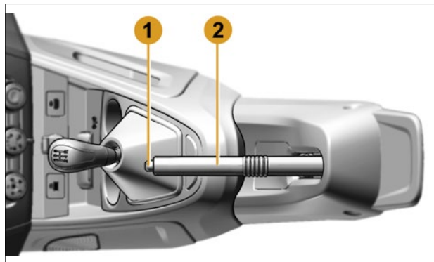
Рис. 3.8.1. Рычаг стояночного тормоза
