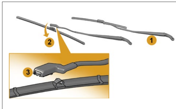
Рис. 6.7.2. Замена щеток стеклоочистителя ветрового стекла
