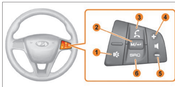
Рис. 3.11.1. Органы управления мультимедийным оборудованием на рулевом колесе
