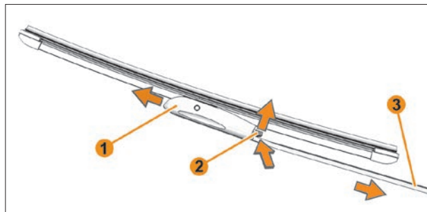
Рис. 9.1. Щетки стеклоочистителя ветрового стекла
