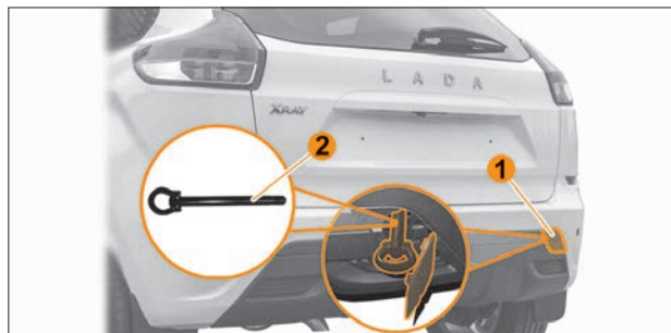
Рис. 9.7. Расположение задней буксирной проушины (в варианте исполнения)
