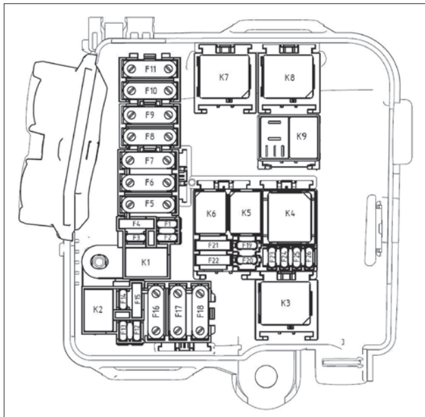
Рис. 8.28. Блок предохранителей и реле моторного отсека
