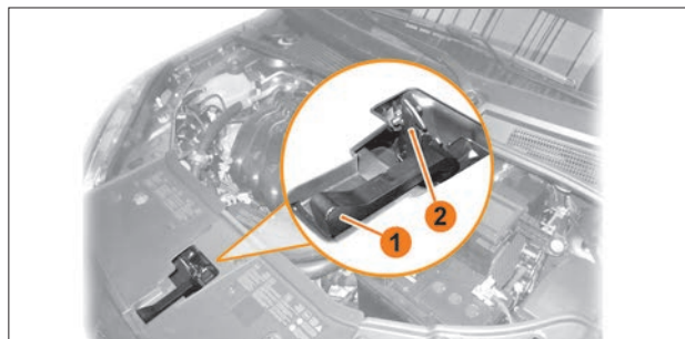
Рис. 8.2. Открытие капота
