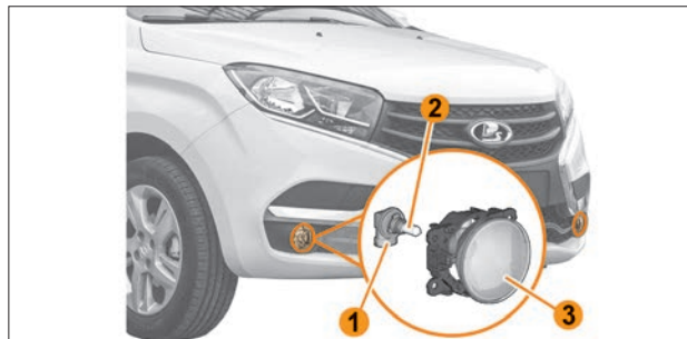
Рис. 8.25. Противотуманная фара
