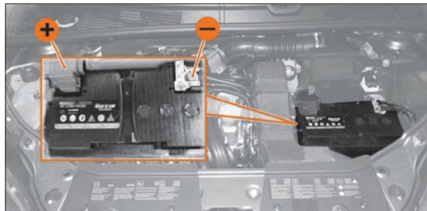
Рис. 8.9. Аккумуляторная батарея
