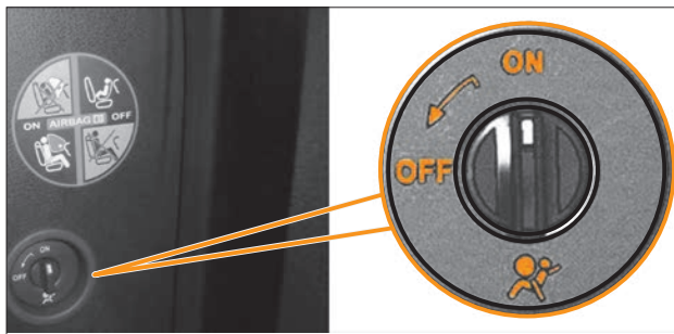
Рис. 2.16. Выключатель подушки безопасности пассажира
