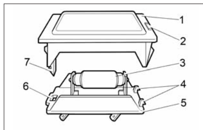
Рис. 63а. Плафон освещения багажника автомобиля с кузовом «седан»
