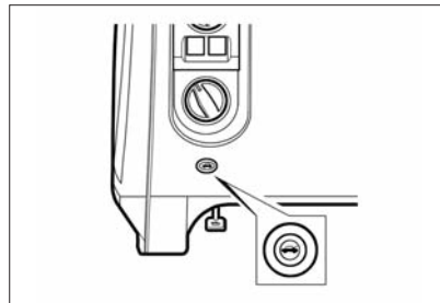
Рис. 26а. Выключатель привода замка багажника (в вариантном исполнении)
