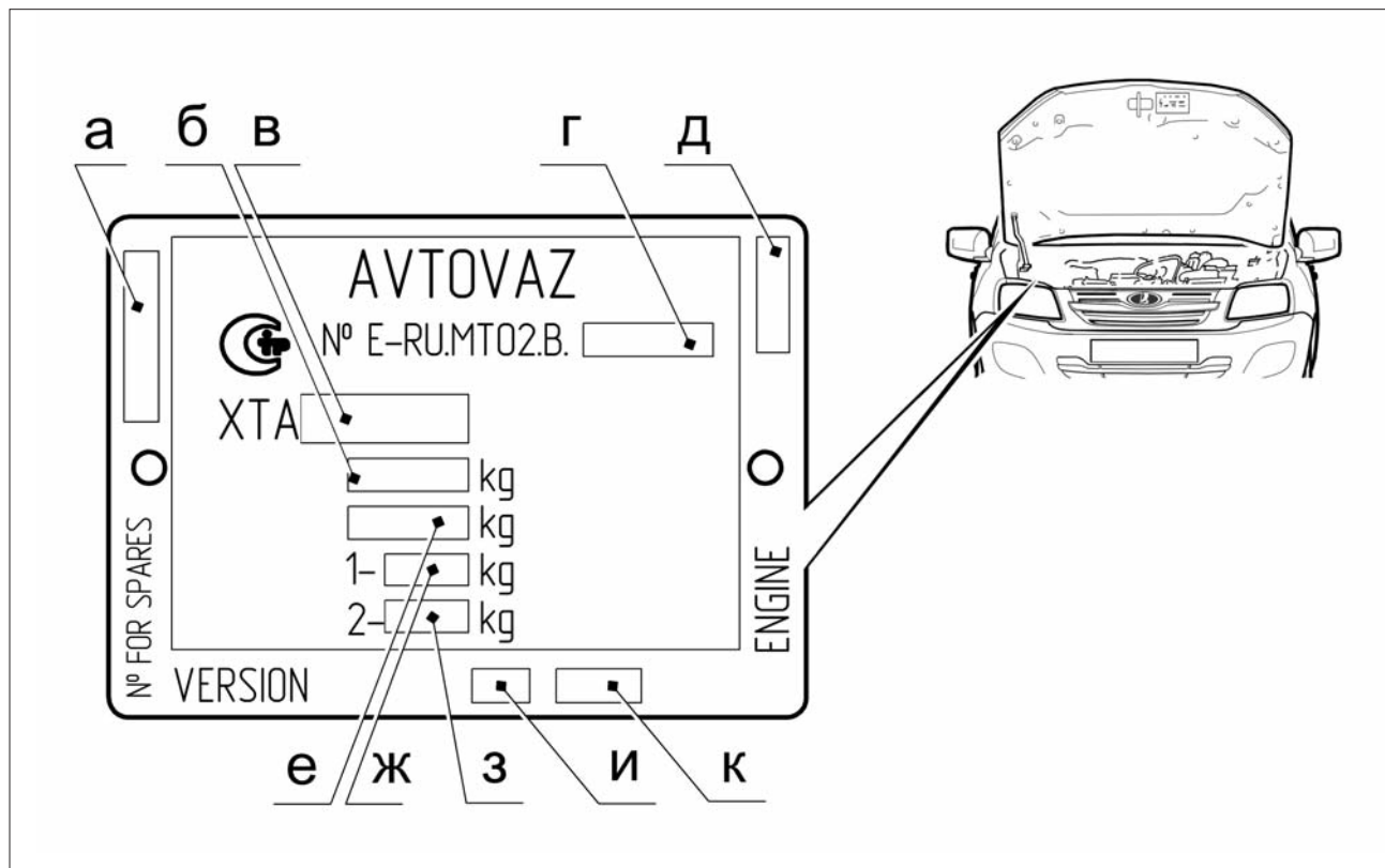
Рис. 66. Паспортные данные
