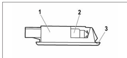
Рис. 63б. Плафон освещения багажника автомобиля с кузовом «лифтбек»
