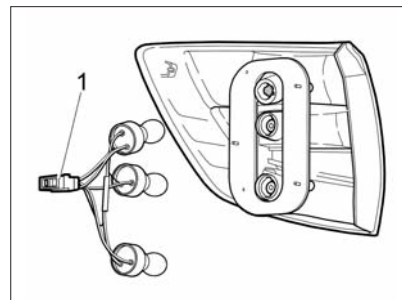
Рис. 60а. Задний фонарь автомобиля с кузовом «седан»
