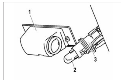
Рис. 61а. Фонарь освещения номерного знака автомобиля с кузовом «лифтбек»
