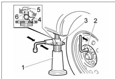
Рис. 536. Подъем автомобиля при замене колес
