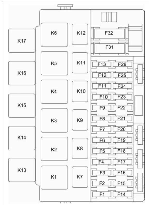
Рис. 58. Блок предохранителей и реле салона ф. АВАР
