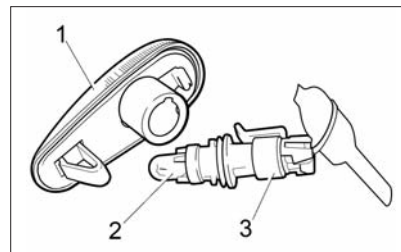
Рис. 60г. Боковой указатель поворота
