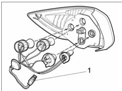
Рис. 60б. Задний фонарь автомобиля с кузовом «лифтбек»
