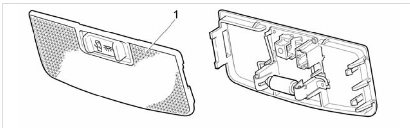
Рис. 62. Плафон освещения салона
