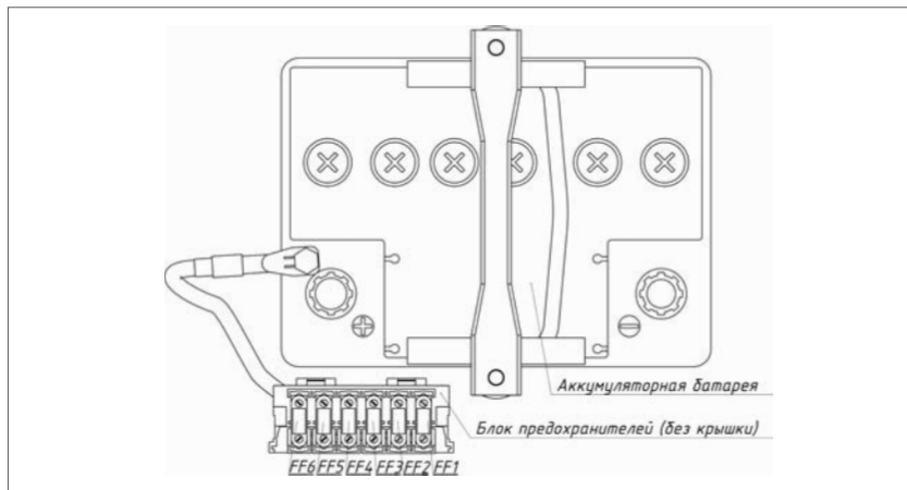
Рис. 57. Блок предохранителей моторного отсека
