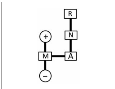
Рис. 48. Схема рычага переключения передач
