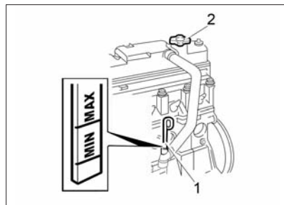
Рис. 45. Проверка уровня масла в картере двигателя 8-клапанного двигателя
