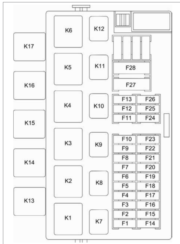
Рис. 59. Блок предохранителей и реле салона ф. DELPHI
