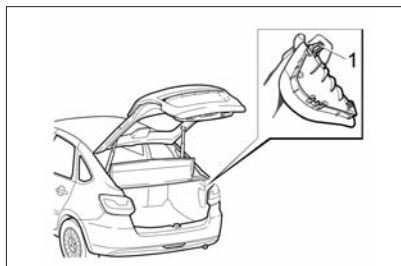
Рис. 59в. Снятие заглушки опоры полки
