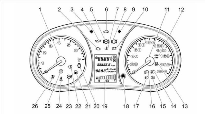
Рис. 29. Комбинация приборов
