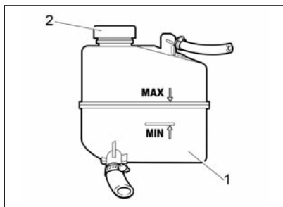
Рис. 46. Расширительный бачок
