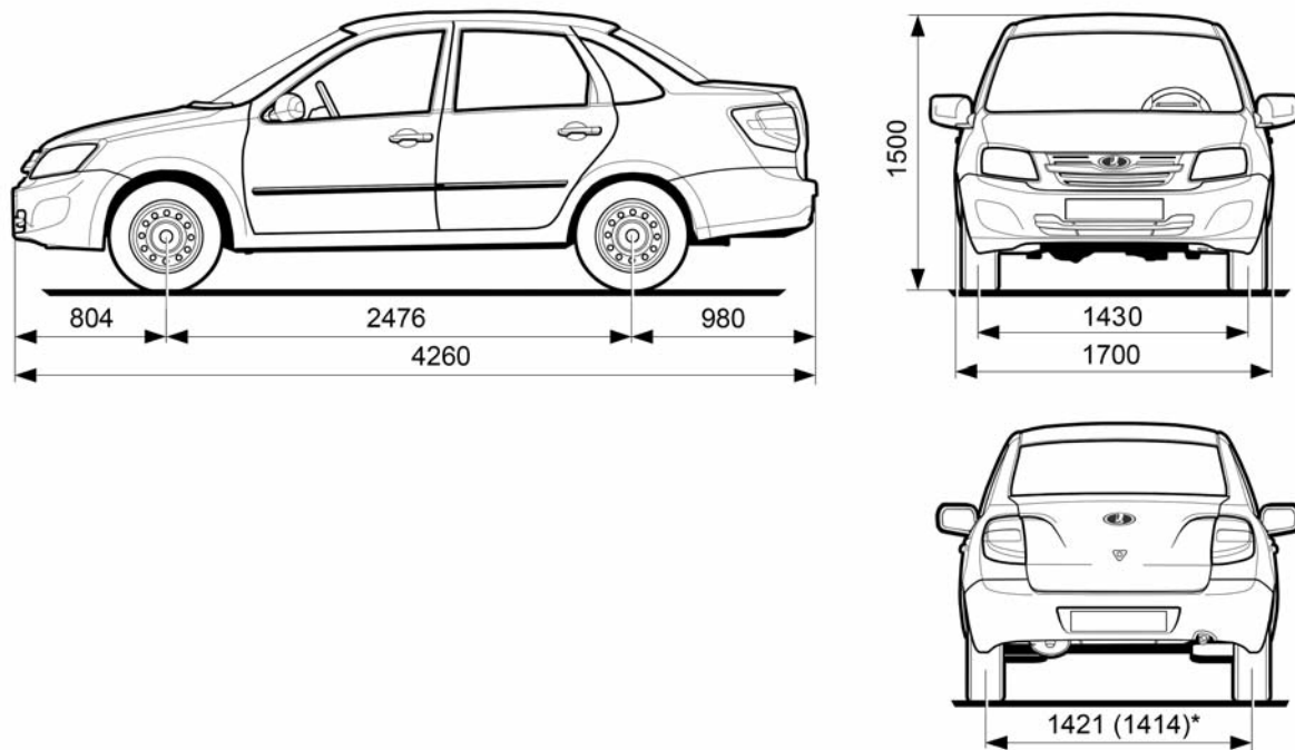
Рис. 64а. Габаритные (справочные) размеры автомобиля 2190 (седан)
