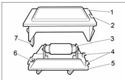
Рис. 62а. Плафон освещения багажника автомобиля с кузовом «седан»
