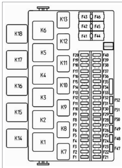
Рис. 57. Монтажный блок
