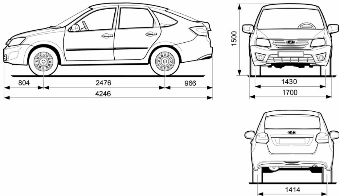
Рис. 646. Габаритные (справочные) размеры автомобиля 2191 (лифтбек)
