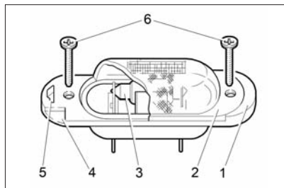
Рис. 60. Фонарь освещения номерного знака автомобиля с кузовом «седан»
