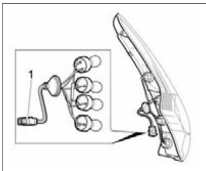
Рис. 60а. Задний фонарь на автомобиле с кузовом «хэтчбек»
