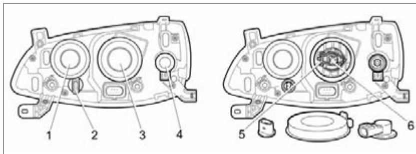
Рис. 59. Блок-фара
