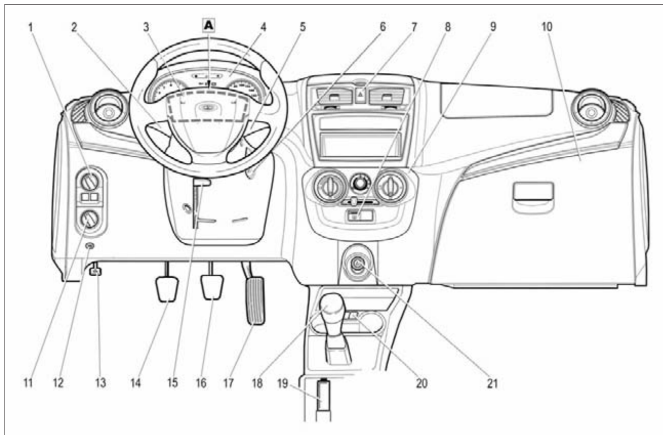
Рис. 30а. Органы управления и приборы (в вариантном исполнении)
