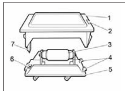
Рис. 65. Плафон освещения багажника и бокового вещевого ящика
