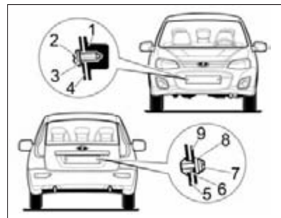
Рис. 45. Крепление номерных знаков
