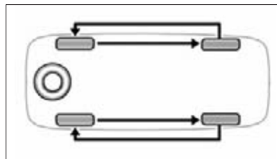
Рис. 54. Схема перестановки колес
