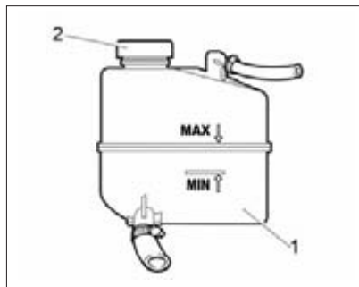
Рис. 50. Расширительный бачок
