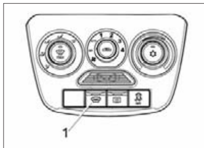
Рис. 43. Выключатель электрообогрева ветрового стекла (в вариантном исполнении)
