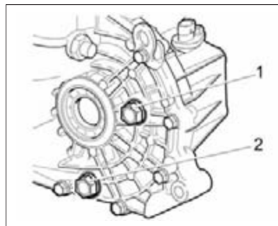
Рис. 49. Проверка уровня масла в механической коробке передач
