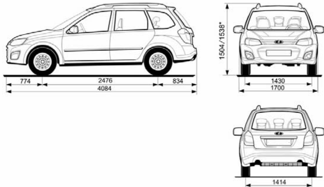
Рис. 68. Габаритные (справочные) размеры автомобиля с кузовом «универсал»
