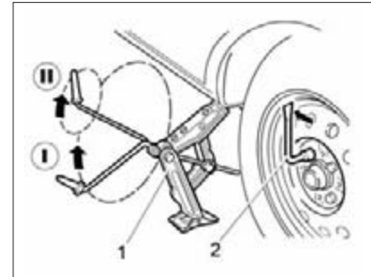
Рис. 55. Подъем автомобиля при замене колес
