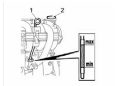
Рис. 48б. Проверка уровня масла в картере 16-клапанного двигателя
