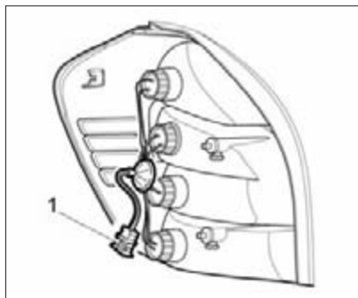
Рис. 60б. Задний фонарь на автомобиле с кузовом «универсал»
