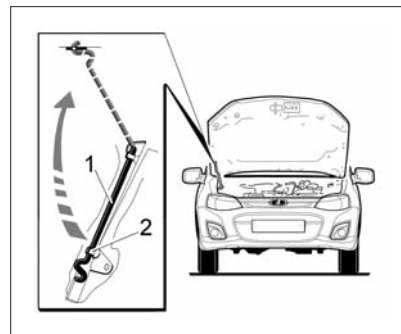
Рис. 26. Открывание капота
