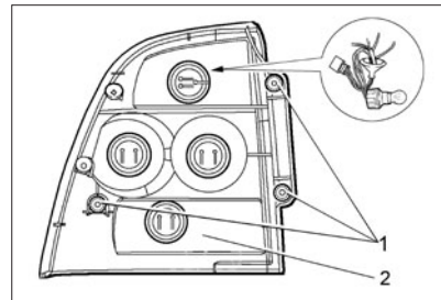
Рис. 88. Задний фонарь
