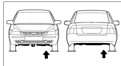
Рис. 43. Буксирование автомобиля
