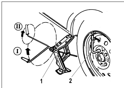
Рис. 53. Замена колес
