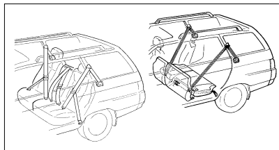
Рис. 11. Положение ремней безопасности при раскладке задних сидений
