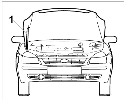
Рис. 28. Установка капота
