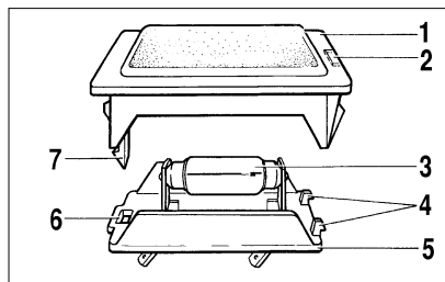
Рис. 63. Плафон освещения вещевого ящика
