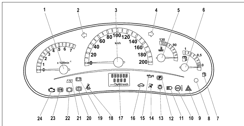
Рис. 32. Комбинация приборов
