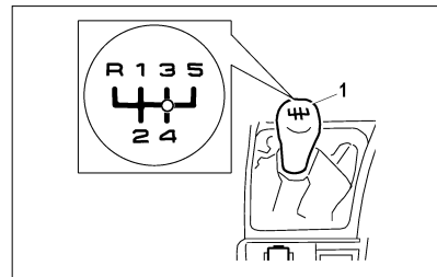
Рис. 38. Рычаг переключения передач
