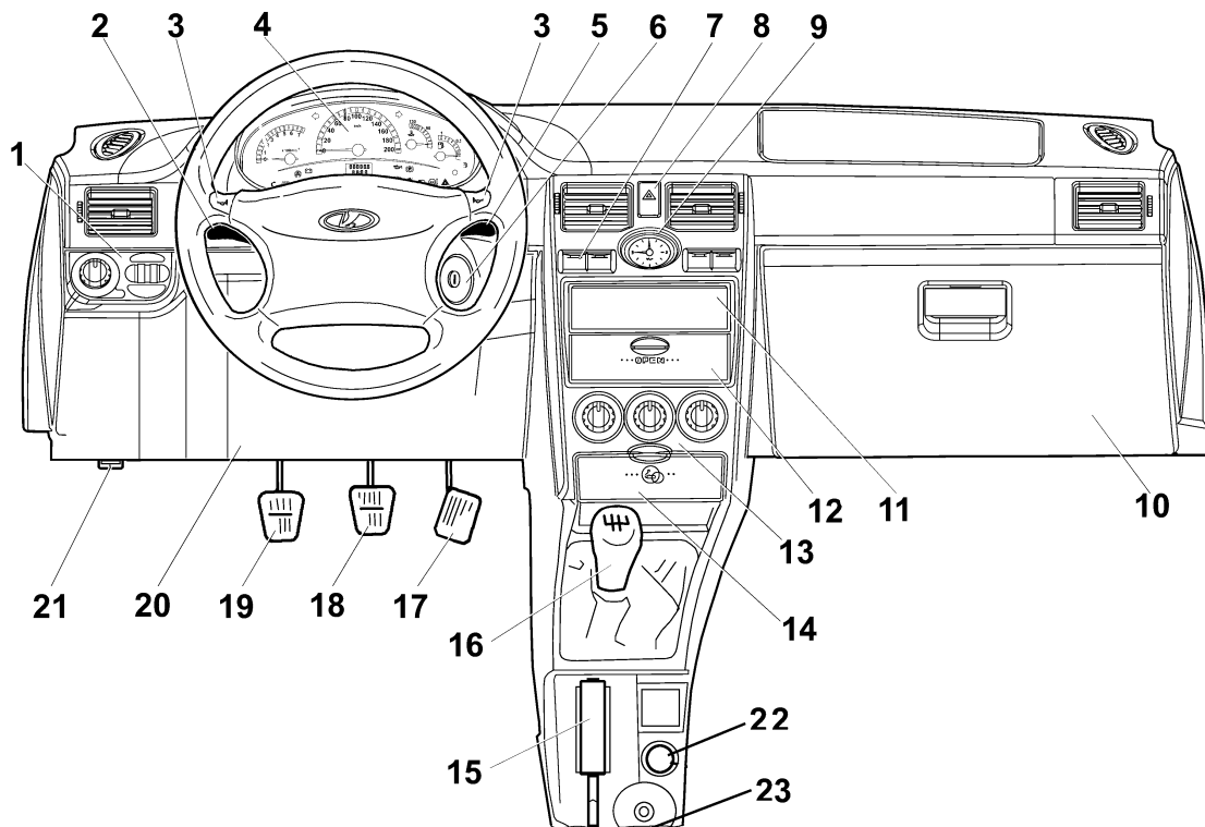
Рис. 31. Органы управления и приборы
