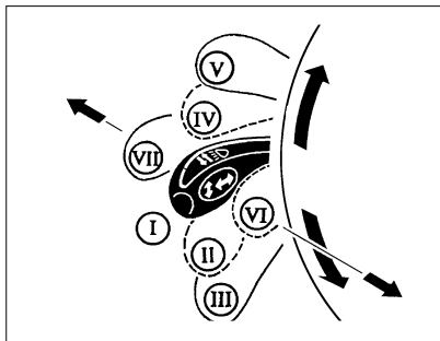
Рис. 35. Переключатель световой сигнализации
