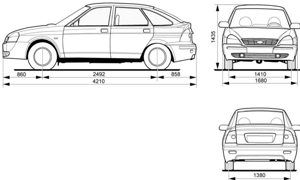
Рис. 65. Габаритные размеры (справочные) автомобиля LADA Priora хэтчбек
