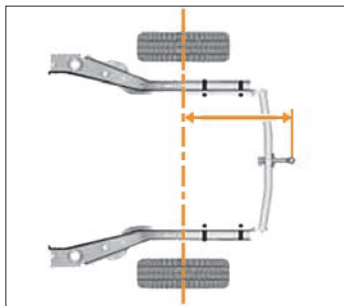
Рис. 9.9. Тягово-сцепное устройство
