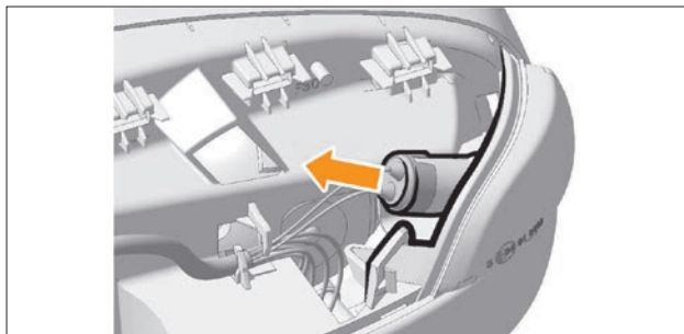
Рис. 8.20. Извлечение патрона
